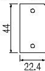
ラックマウント 連結パネルA 1個
